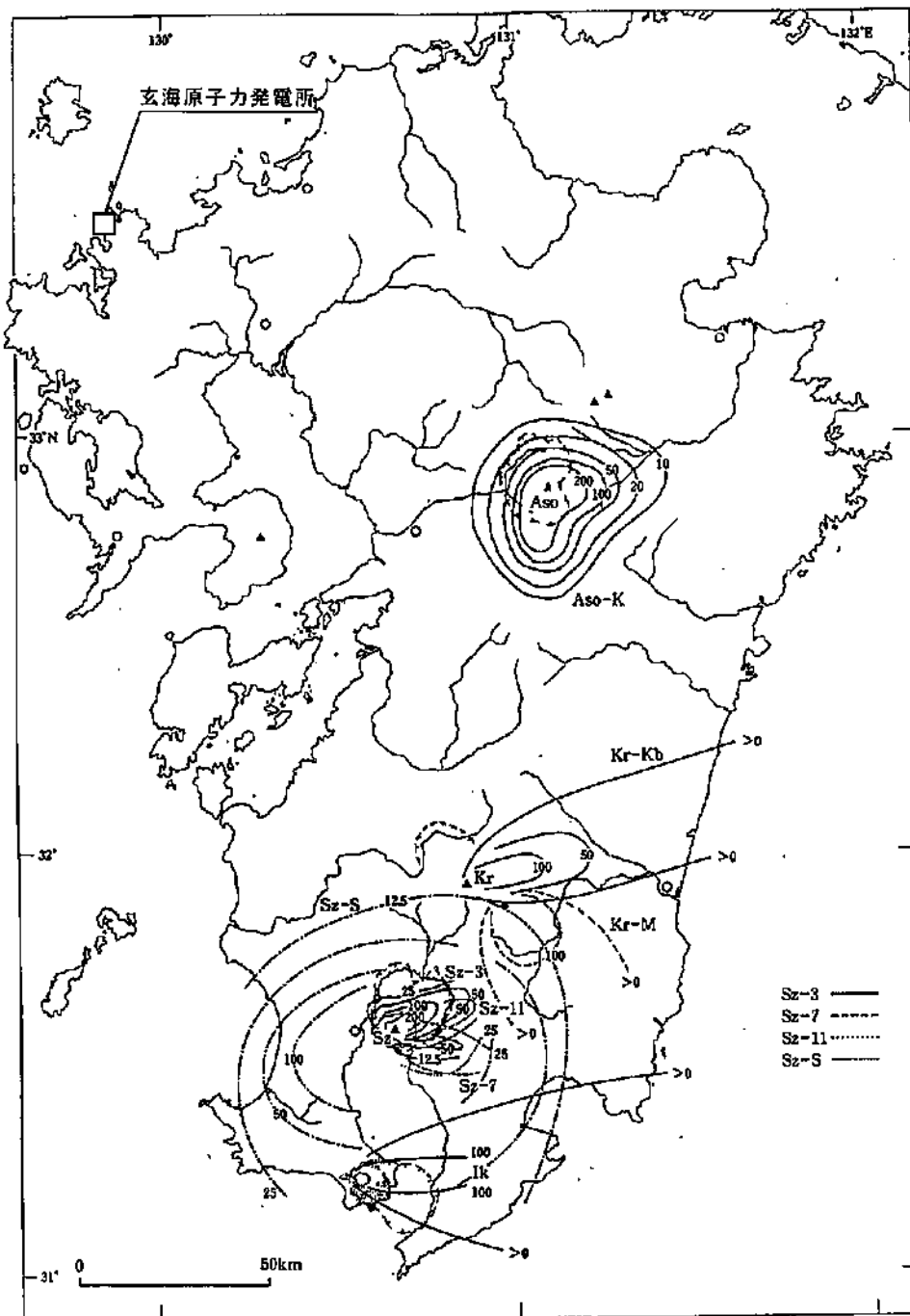
図 3.1-1 九州地方の約 3 万年前以降の主要テフラの等層厚線図。
