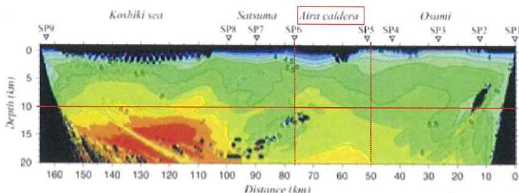
図8 宮町ほか(2018)【乙イ B112】で示されている二次元P波速度構造 7
