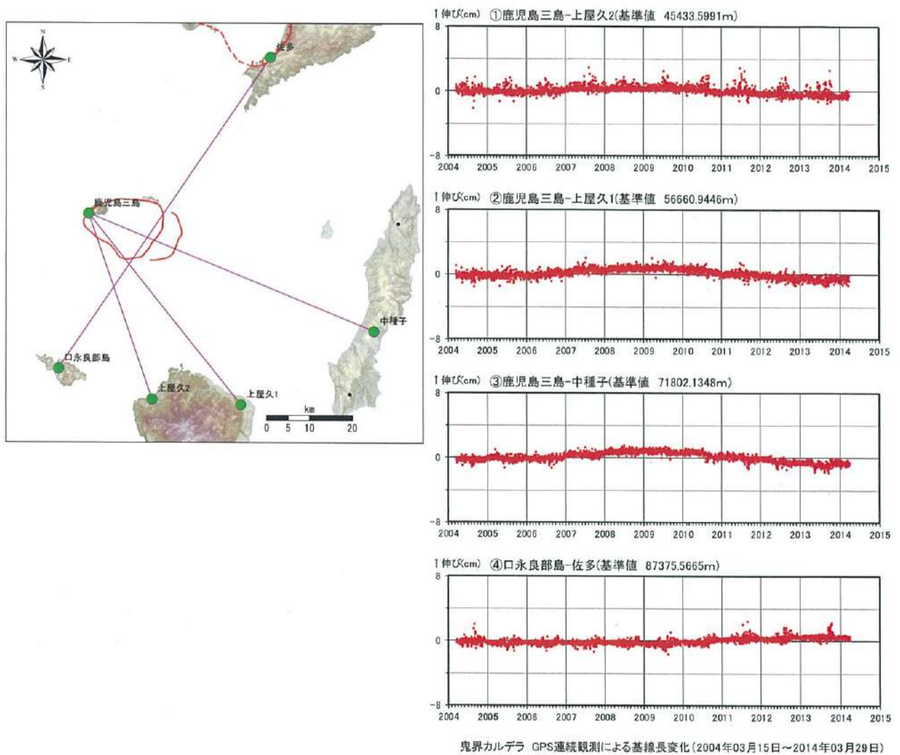
図17 鬼界カルデラにおけるGPS観測結果 12
