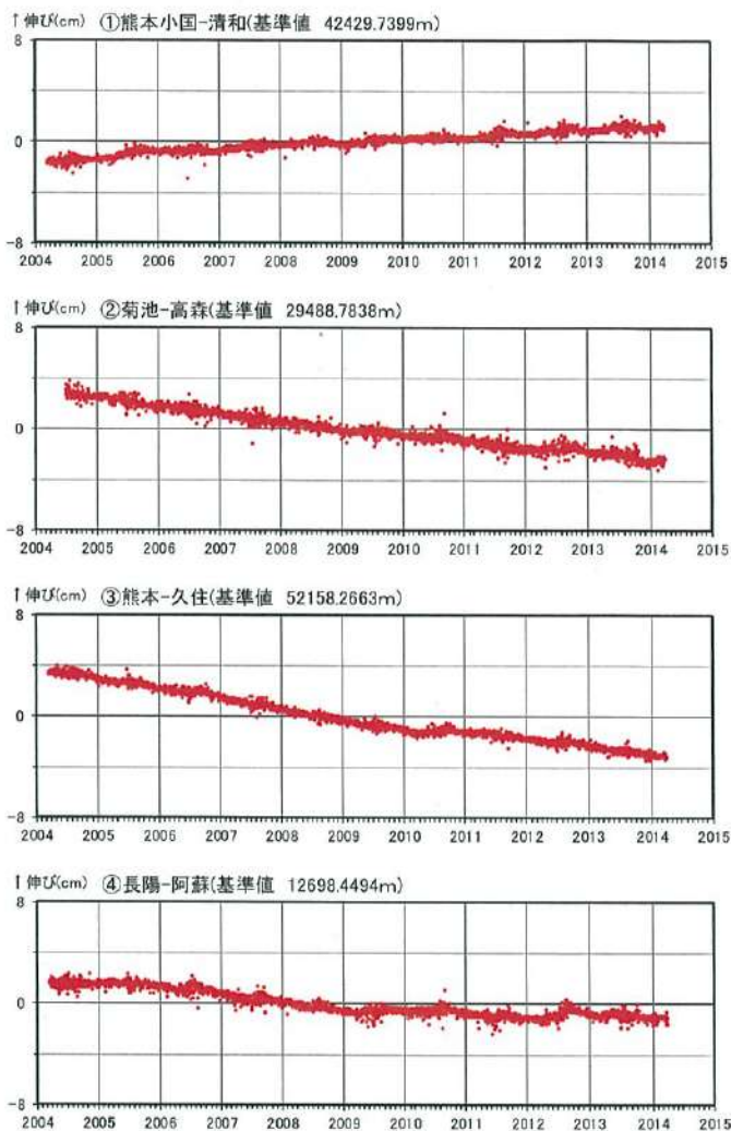
阿蘇カルデラ GPS連続観測による基線長変化(2004年03月15日～2014年03月29日)
