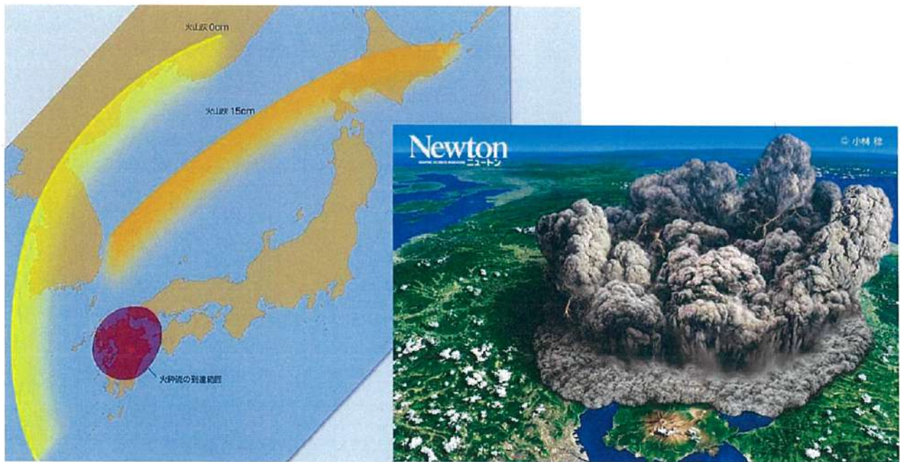
図2 破局的噴火の影響及びイメージ図
